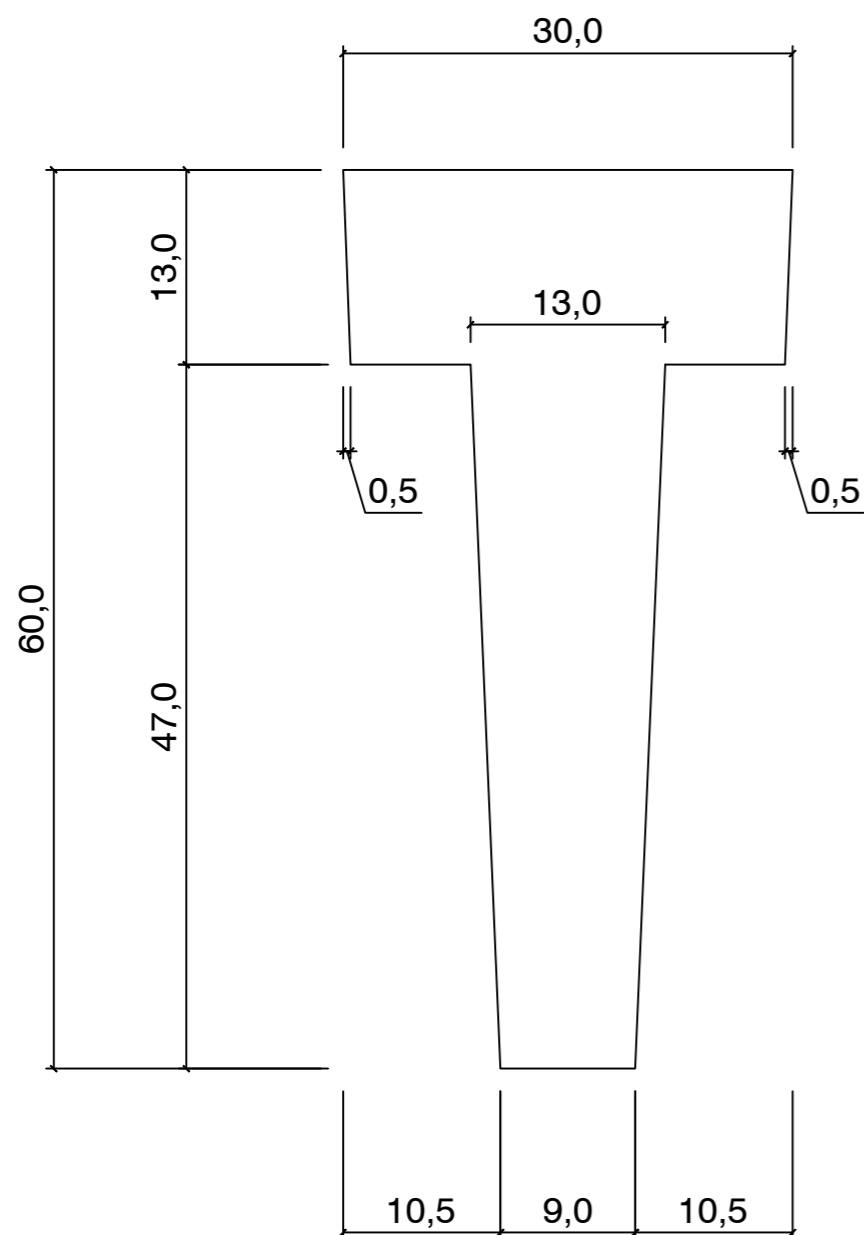
ALZADO PIEZA VT-60
